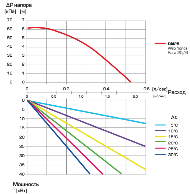
Диаграмма встроенного насоса
